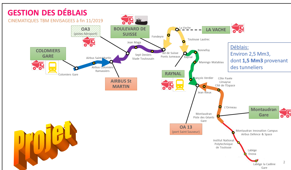
Figure 1: Cinématique de tunnelier envisagée à fin 11/2019
